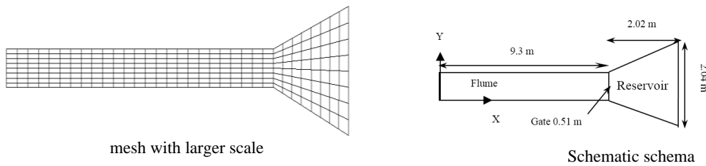
شکل ۵. محدوده مورد مطالعه، مخزن و فلوم مدل آزمایشگاهی میرمحمدحسینی [14].
