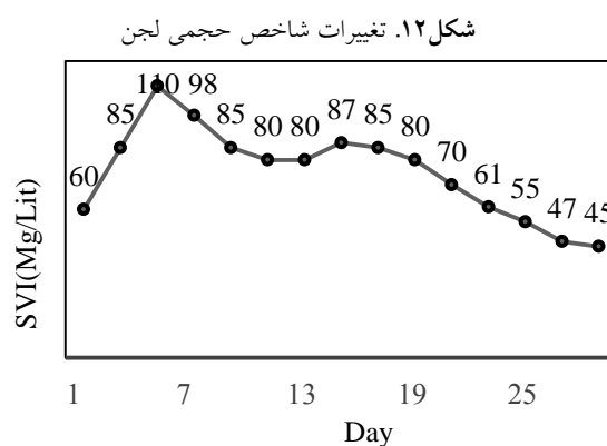
Fig. 12. Sludge volum index changes
